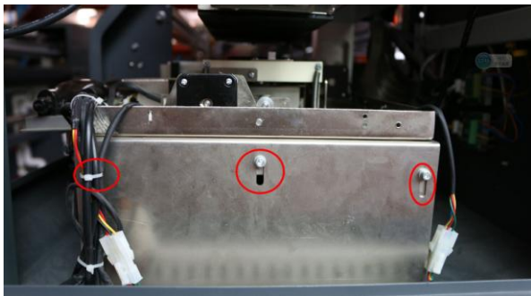
GEN5 墨栈调整上下
