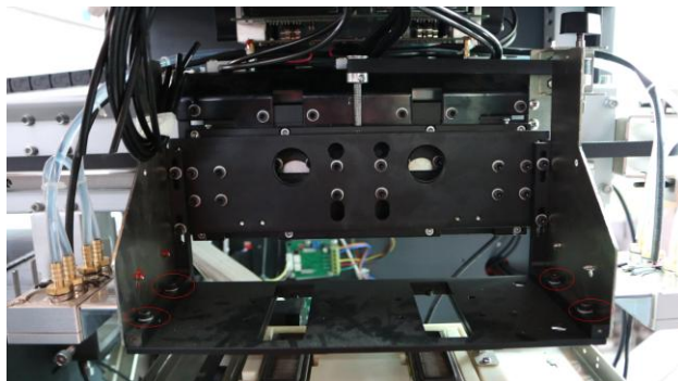
GEN5 喷头的调整位置（红圈）
